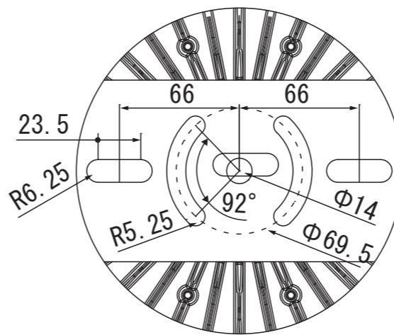
詳細図 A 1 ; 3
